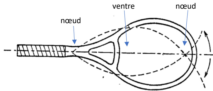
Figure 37 : Nœud et ventre de vibrations lors de la vibration de la raquette dans le plan de la raquette – Schéma issu de la publication [1]
