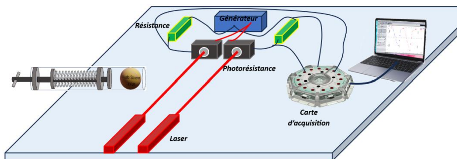
Figure 4 : mesure de la vitesse de la balle à la sortie du lance balle à l'aide de 2 lasers et 2 photorésistances
