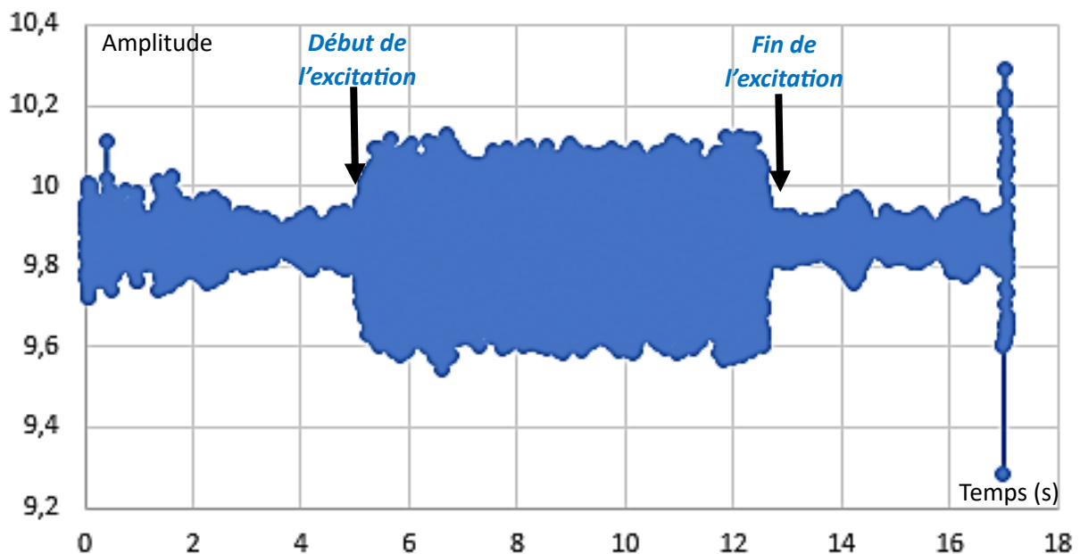
Figure 23 : mesure de la vibration au niveau du manche au moyen d'un accéléromètre posé sur le manche
