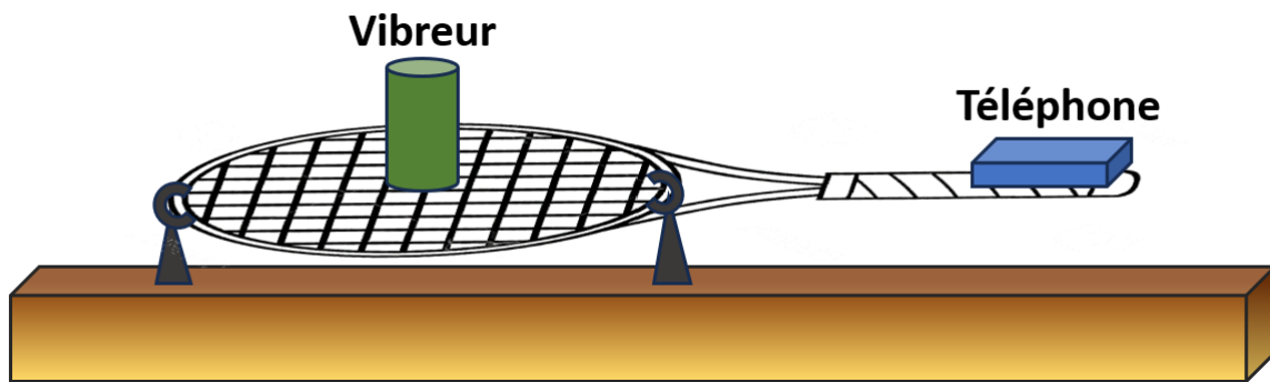
Figure 22 : vibration du manche au moyen d'une membrane vibrante disposée sur le cordage – Mesure de la vibration grâce à l'accéléromètre du téléphone piloté par l'application Phyphox
