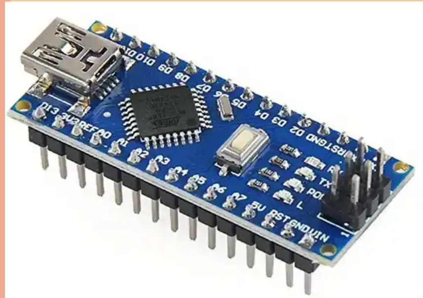
Arduino Nano
